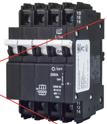
DIN mount 4 Pole + Auxiliary
